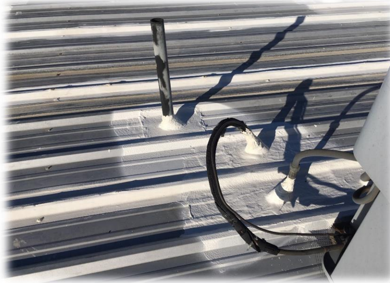
Reinforce Conduit
